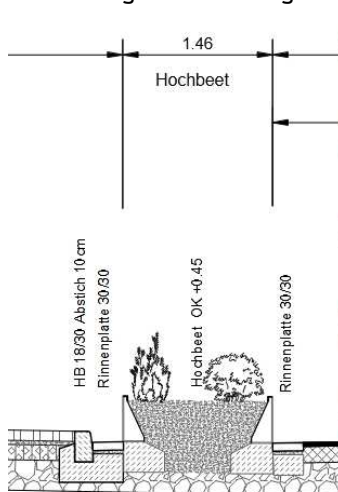
Abb: Querschnitt Anlage Hochbeet
