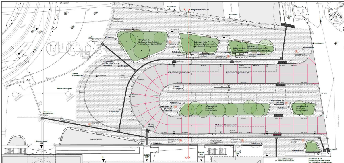
Abb: Planzeichnung
